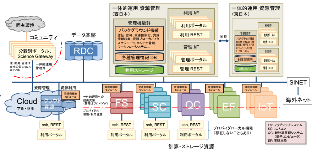
一体的運用計算基盤の構成例
