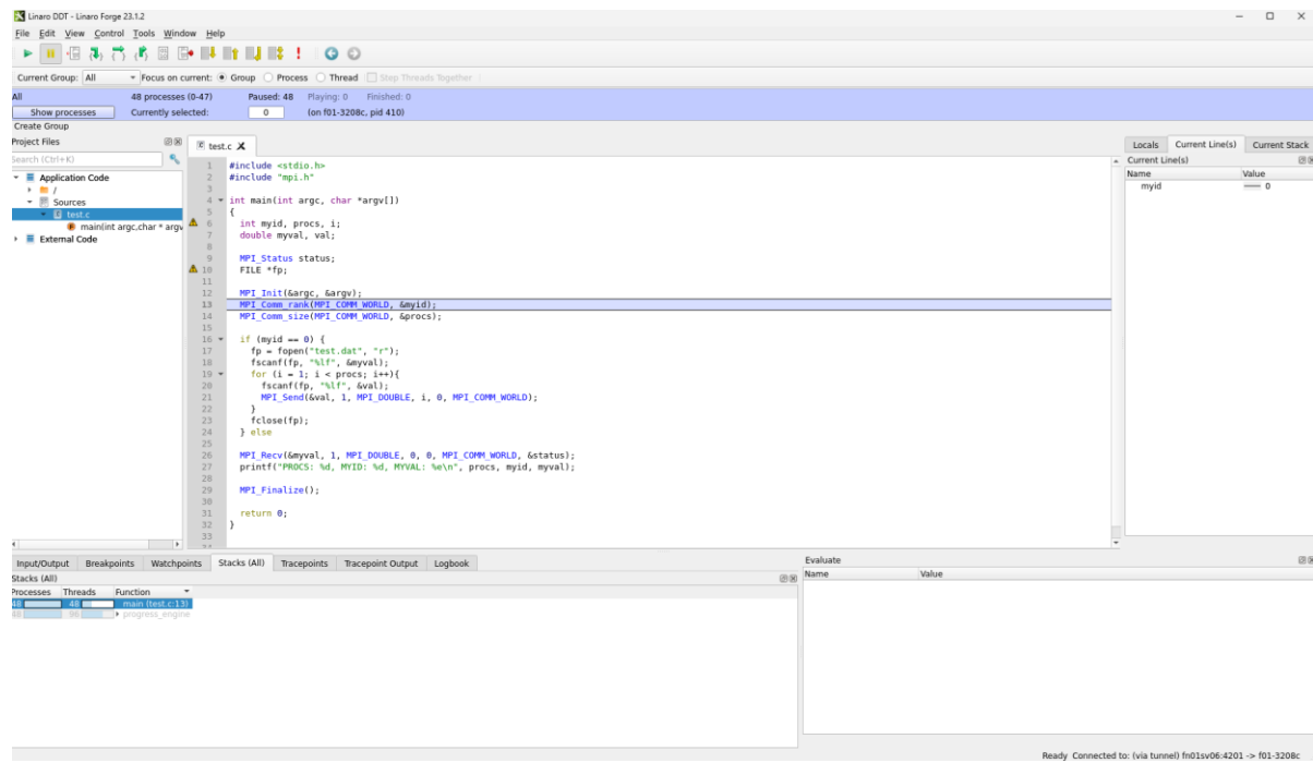
Linaro DDT
