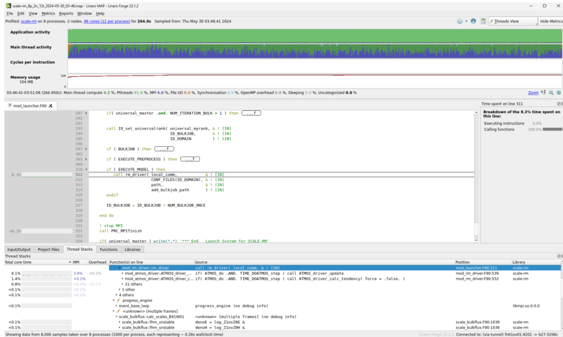
Linaro MAP
