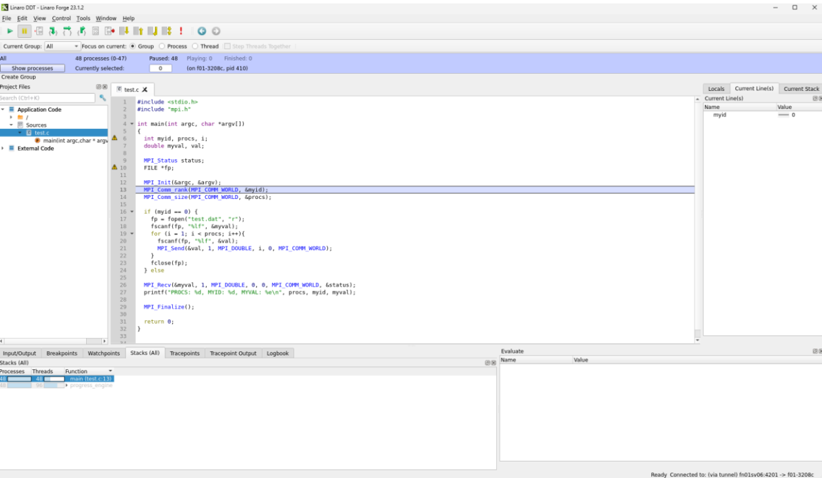
Linaro DDT
