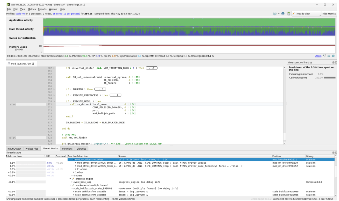
Linaro MAP
